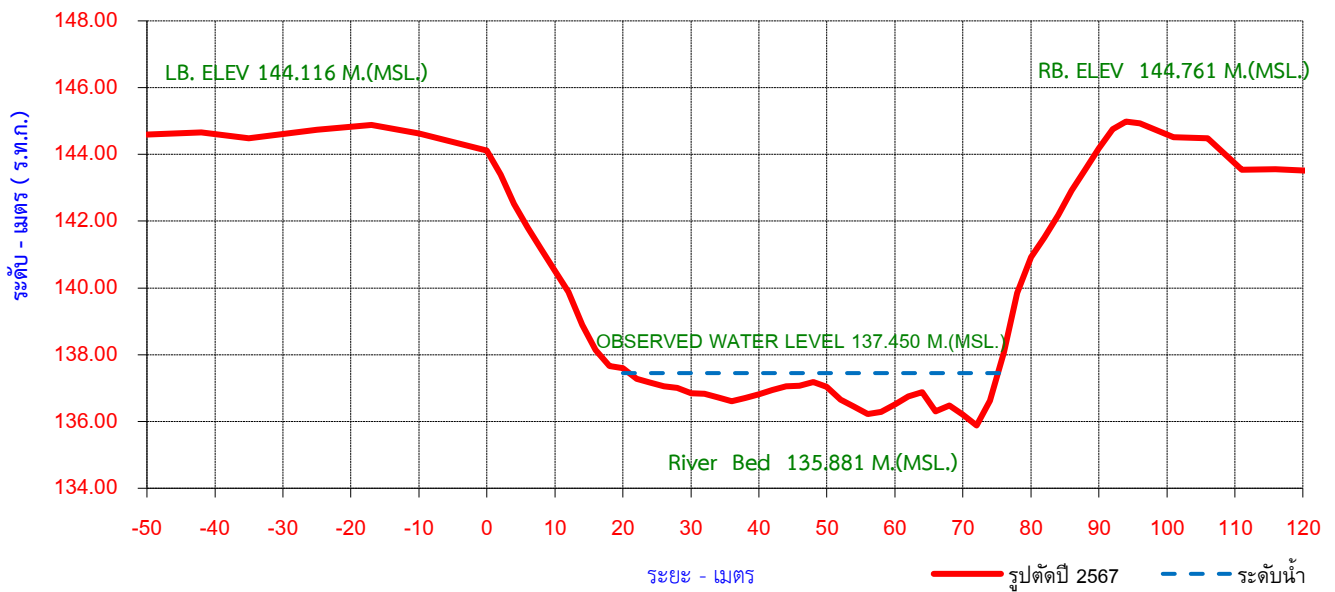
รูปตัดขวางลำน้ำ ปีน้ำ 2567 สถานี W.24 แม่น้ำวัง อ.สามเงา จ.ตาก
